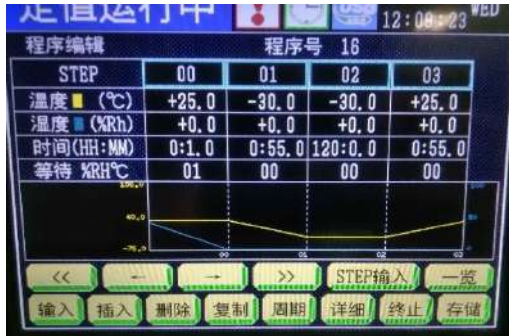
Test program setup 试验程序设置图
