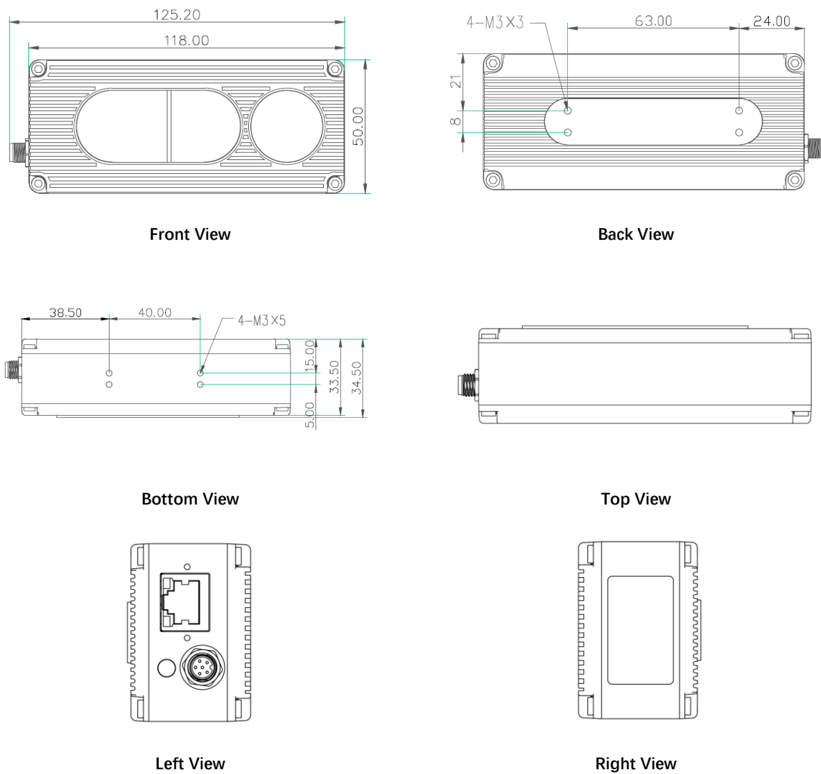
图 3.1: DS86 产品结构 (单位:mm)
